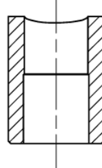
NPTF Gewinde/Thread IG NPTF / AG NPTF
