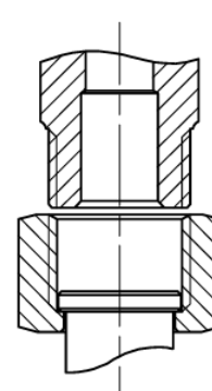
G Gewinde/Thread IG G / AG G
