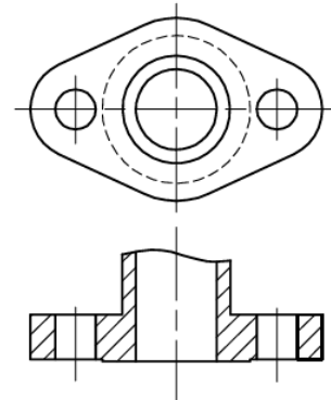
Flanschanschluss Flange connection
