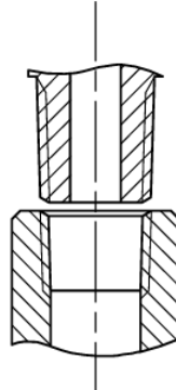
NPTF Gewinde/Thread IG NPTF / AG NPTF
